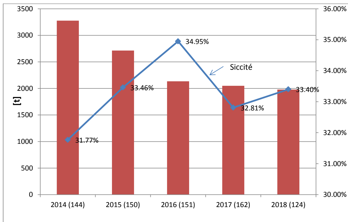
Figure 5 : Tonnage des boues déshydratées évacuées.
