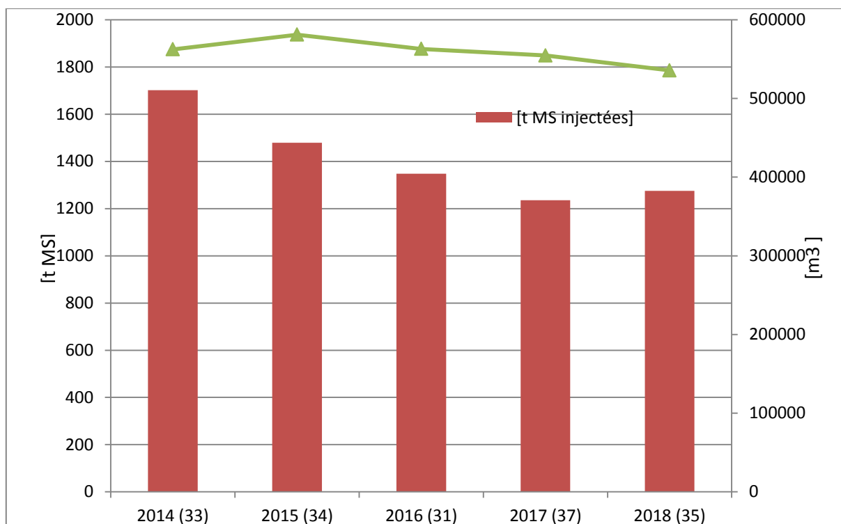
Figure 4 : Tonnage des boues injectées en digestion (en tonnes MS).
