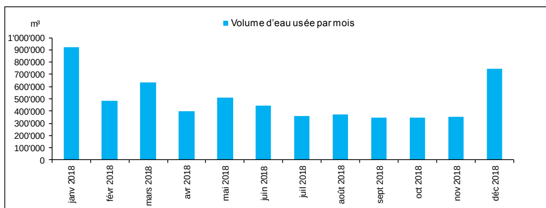
Figure 1 : Volumes mensuels d'eau usée traités par la STEP
