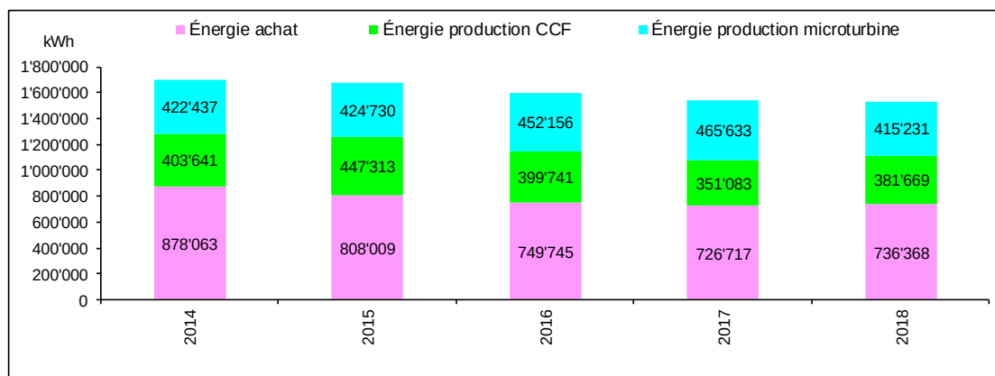
Figure 6 : Bilan électrique.
