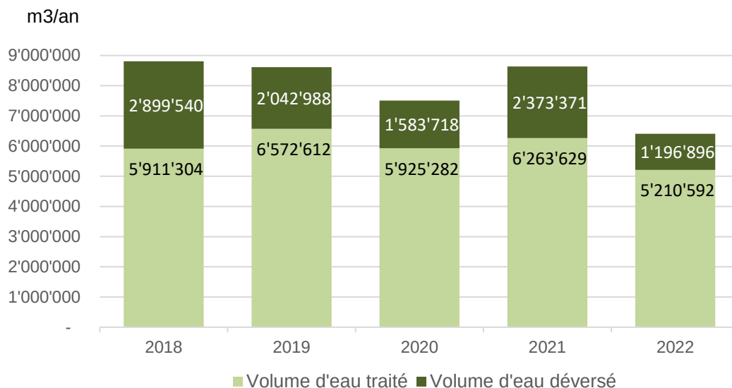
Figure 2 : Volumes annuels d'eaux usées traitées et déversées par la STEP
