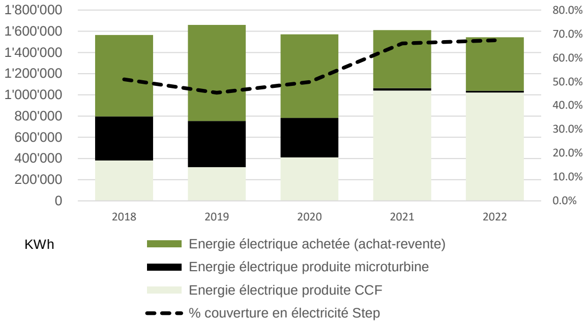
Figure 3 : Bilan électrique
