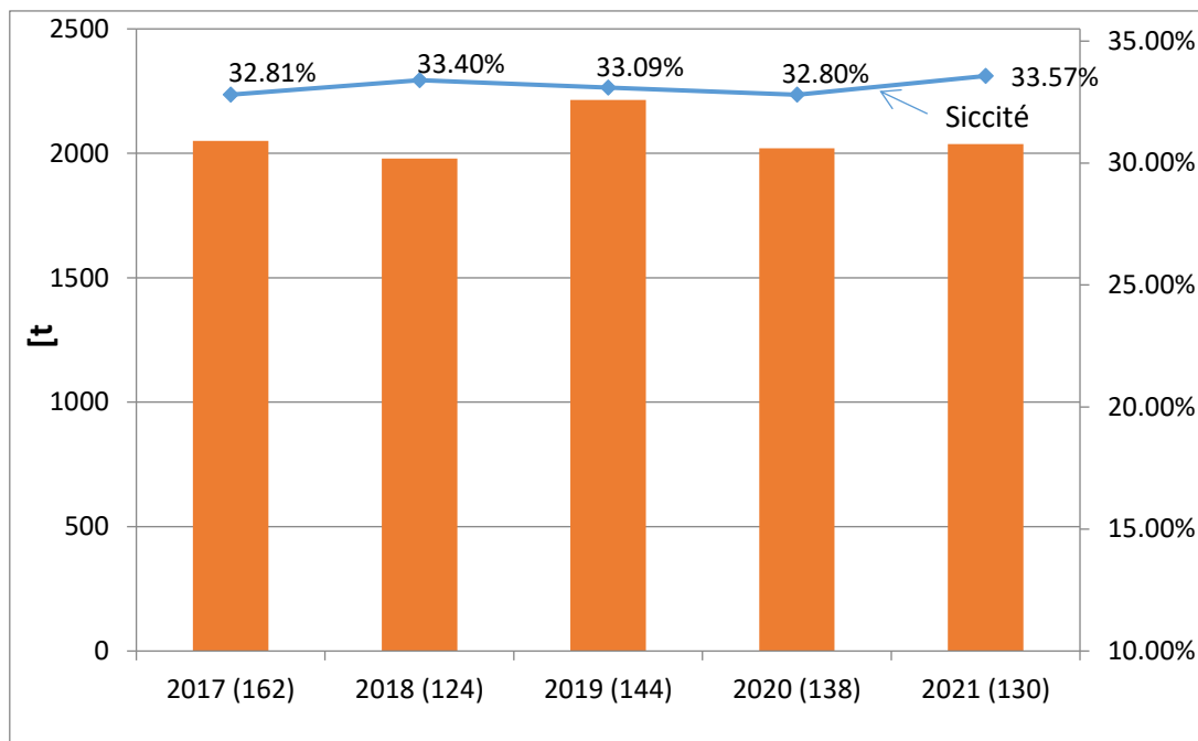
Figure 5 : Tonnage et siccité des boues déshydratées évacuées
