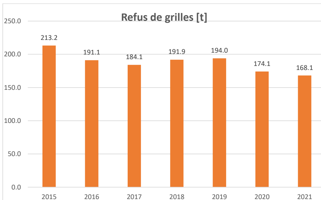
Figure 3 : Déchets de grilles évacués
