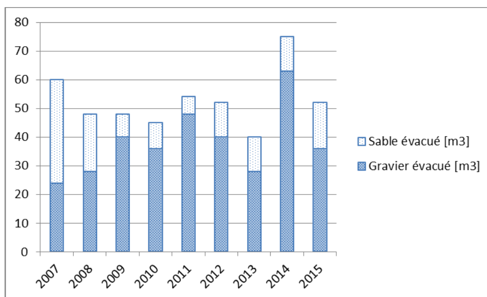
Figure 2 : Sable et gravier évacués
